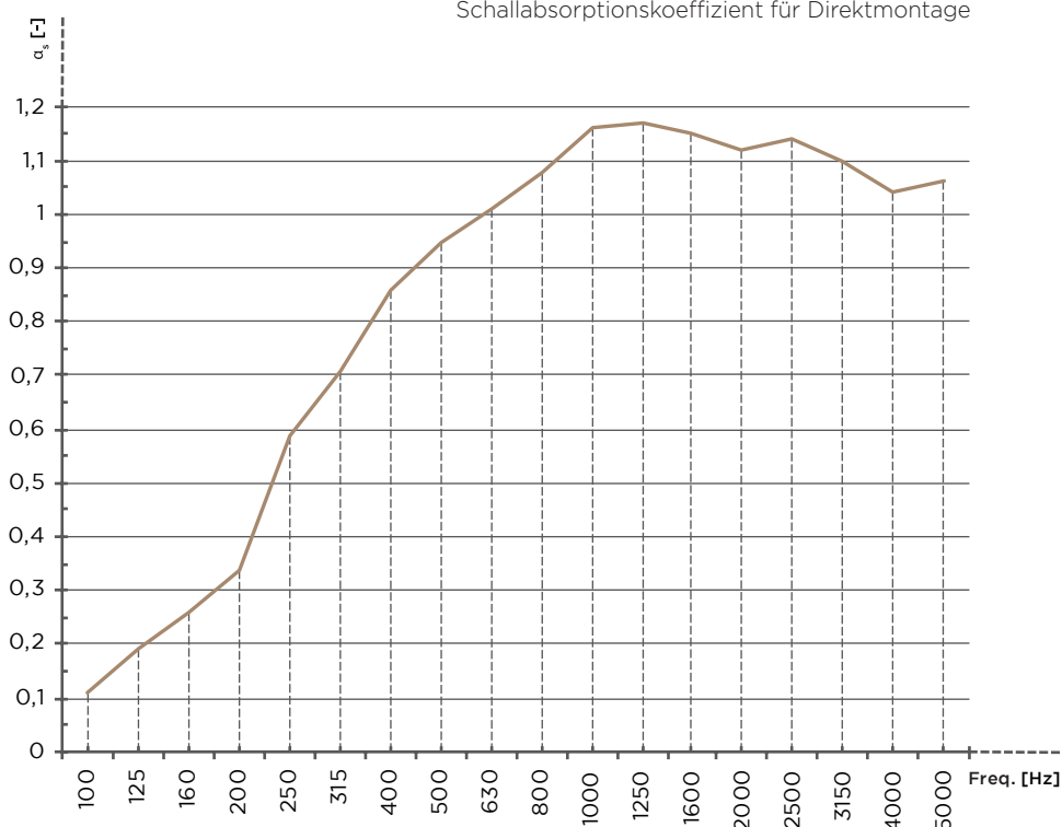
Schallabsorptionskoeffizient für Direktmontage
